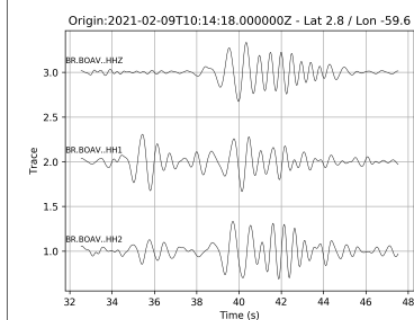
Fig. 2: Template T2, usando 0.9-2.5 Hz S+0 até S+15 segundos.
