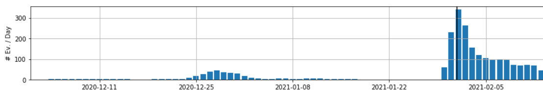
Fig. 12: Distribuição temporal do catálogo gerado pelo template T2 utilizando um limiar de detecção igual a 0.40. Com esse valor é possível dectar um total de 2335 eventos, incluindo o evento principal ocorrido no dia 2021-01-31 às 19:05 UTC.
